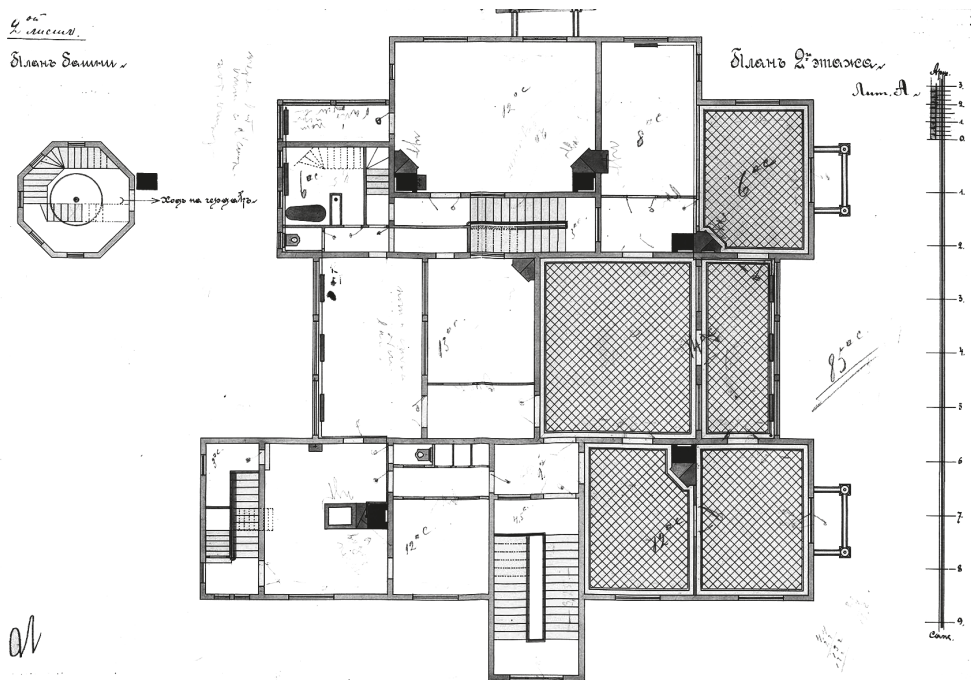
Рис. 3. Проект дома П. А. Авенариуса лит. «А». План 2-го этажа. Копия. 1908. ЦГИА СПб. Ф. 1546. Оп. 5. Д. 1520. Л. 9, 10
