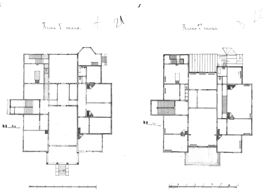
Рис. 9. Проект перестройки дачи М.Ф.Святополк-Мирской (бывшей дачи П. А.Авенариуса). Планы 1-го и 2-го этажей. Архитектор И.П.Володихин. 1914. ЦГИА СПб. Ф. 1546. Оп. 5. Д. 1520. Л. 21, 22
