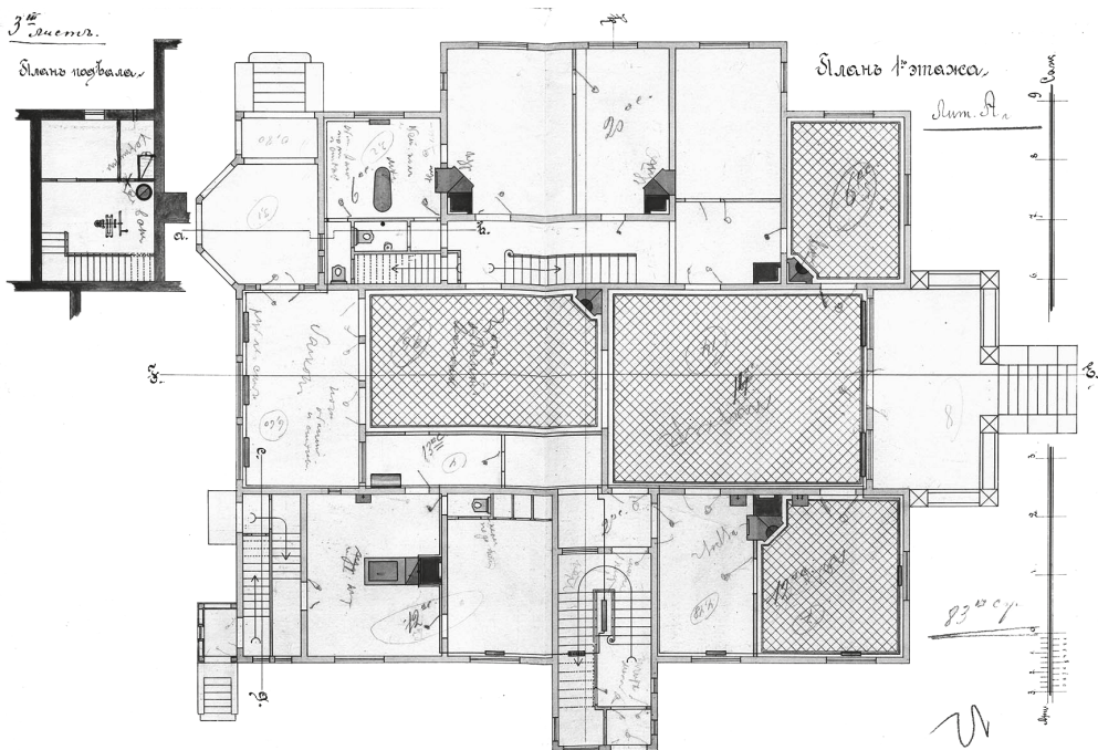
Рис. 2. Проект дома П. А. Авенариуса лит. «А». План 1-го этажа. Копия. 1908. ЦГИА СПб. Ф. 1546. Оп. 5. Д. 1520. Л. 11, 12
