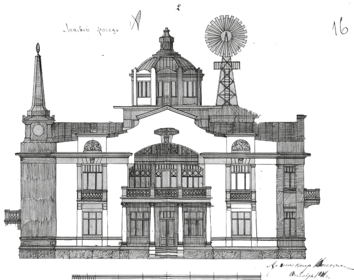
Рис. 7. Проект перестройки дачи М. Ф. Святополк-Мирской (бывшей дачи П. А. Авенариуса). Западный фасад. Архитектор И. П. Володихин. 1914. ЦГИА СПб. Ф. 1546. Оп. 5. Д. 1520. Л. 16
