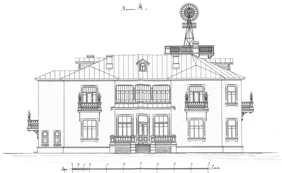
Рис. 4. Проект дома П. А. Авенариуса лит. «А». Западный фасад. Копия. 1908. ЦГИА СПб. Ф. 1546. Оп. 5. Д. 1520. Л. 30, 31
