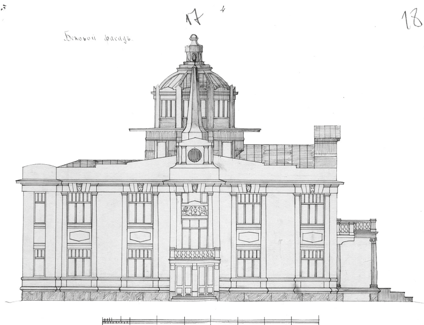
Рис. 8. Проект перестройки дачи М. Ф. Святополк-Мирской (бывшей дачи П. А. Авенариуса). Северный фасад. Архитектор И. П. Володихин. 1914. ЦГИА СПб. Ф. 1546. Оп. 5. Д. 1520. Л. 17, 18
