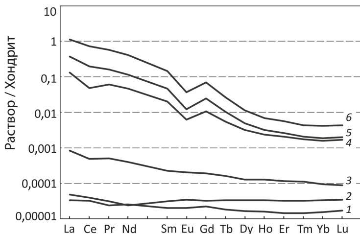
Рис. 4. Распределение редкоземельных элементов при взаимодействии глинистой фракции пещерных осадков и экспериментальных растворов с различными значениями рН (1–3) и при выщелачивании гранитидов кислотными растворами в окислительной атмосфере (4–6):
