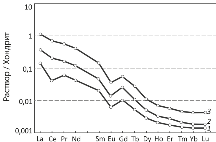
Рис. 3. Распределение редкоземельных элементов в экспериментальных растворах по выщелачиванию гранитоидов в кислых окислительных условиях в зависимости от времени взаимодействия: 1 — 10 мин, 2 — 1 сут, 3 — 4 сут
