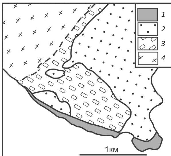
Рис. 2. Геологическое строение западного берега оз. Мало-го Янисъярви:
