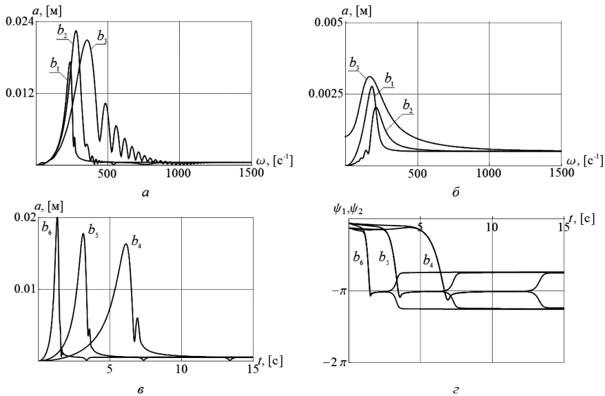
Рис. 4. Прохождение критической области при различных значениях углового ускорения b : b_1 = 0.25 \text{ c}^{-2} , b_2 = 2.5 \text{ c}^{-2} , b_3 = 12.5 \text{ c}^{-2} , b_4 = 0.04 \text{ c}^{-2} , b_5 = 0.08 \text{ c}^{-2} и b_6 = 0.2 \text{ c}^{-2} .
