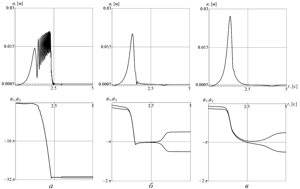
Рис. 5. Влияние коэффициента демпфирования в АБУ: c_\psi = 0.01 \text{ кг/с}\cdot\text{м}^2 (а); c_\psi = 0.1 \text{ кг/с}\cdot\text{м}^2 (б); c_\psi = 0.4 \text{ кг/с}\cdot\text{м}^2 (в).
