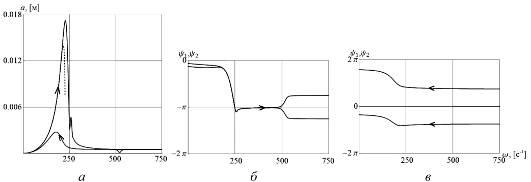
Рис. 3. Прямое и обратное прохождения критической области с постоянным угловым ускорением в случае, когда масса шариков достаточна для балансировки.
