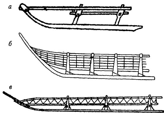
Рис. 4. Ручные нарты.
