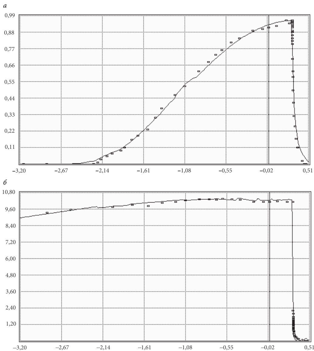
Рис. 5. График временного прослеживания S\text{-}lg t понижения-восстановления уровня а — по наблюдательной скважине 76; б — по центральной скважине 72.
