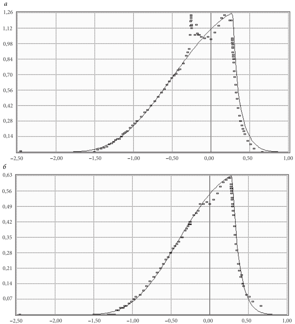
Рис. 7. Графики временного прослеживания понижения-восстановления уровня по скважинам (начало рисунка):
