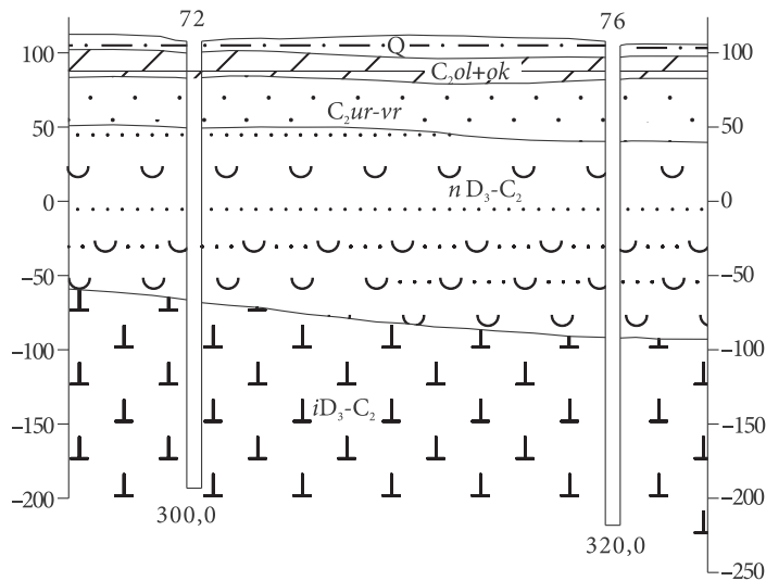
Рис. 4. Схематический геологический разрез по линии скважин опытного куста 72–76
