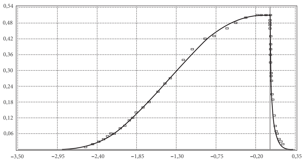
Рис. 3. График временного прослеживания S\text{-}lg t понижения-восстановления уровня по наблюдательной скважине 107^B
