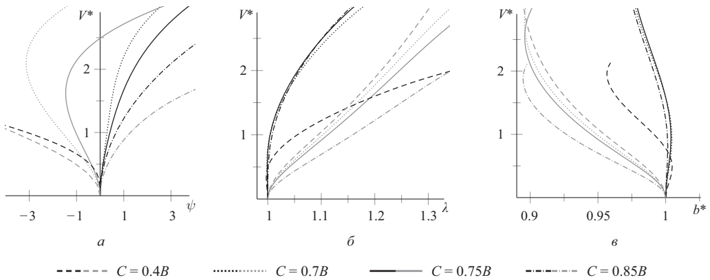
Рис. 2. Зависимость между безразмерным электрическим напряжением V^* и углом закручивания \psi (в градусах) (а), кратностью удлинения \lambda (б), относительным внешним радиусом b^* (в) при A = 0.2B для разных значений C ; углы намотки \Phi_1 = 3\pi/4 , \Phi_2 = \pi/4 . Черные линии — напряжение прикладывается к внутреннему слою (электроды A и C ). Серые линии — напряжение прикладывается к внешнему слою (электроды C и B ).
