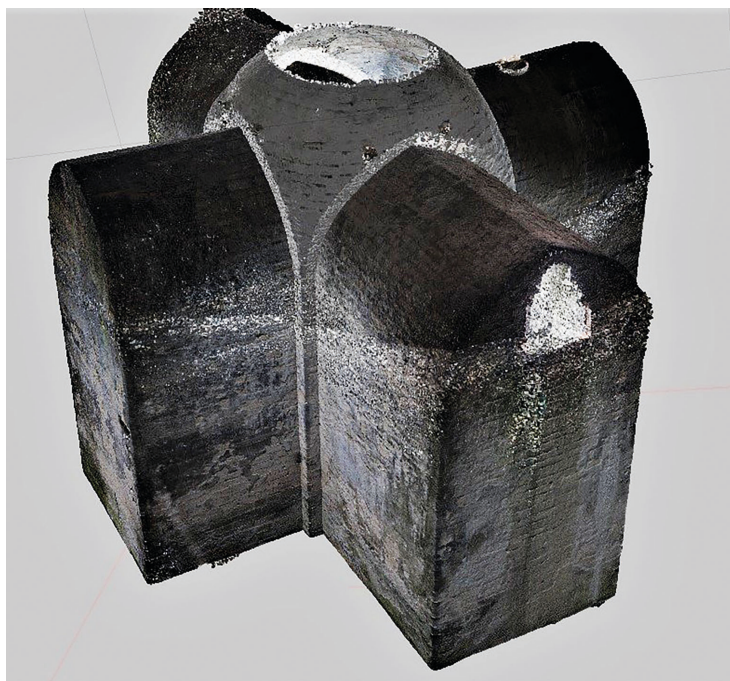
Рис. 10. Фотограмметрическая 3D-модель храма. Фото Д. Л. Шишкова
