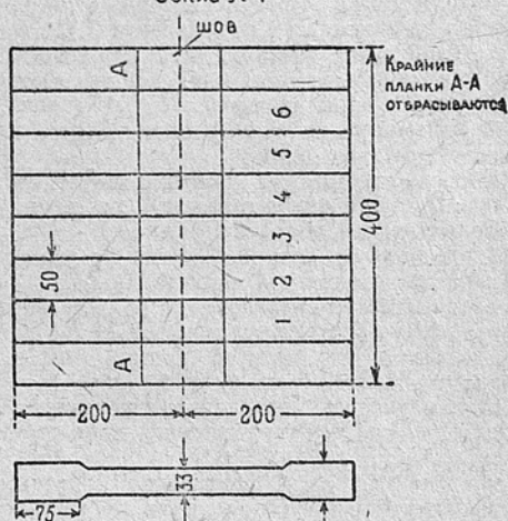
ФОРМА ПЛАНКИ ДЛЯ ИСПЫТАНИЯ НА РАЗРЫВ
