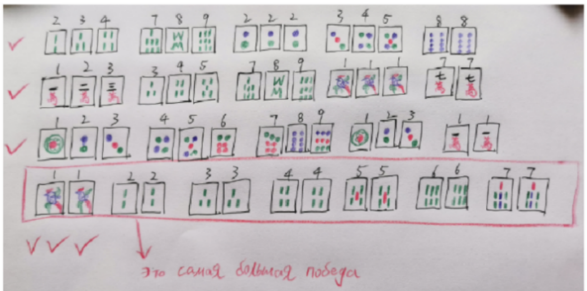
Рис 1.1.2 Иллюстрация метода победы в маджонге
