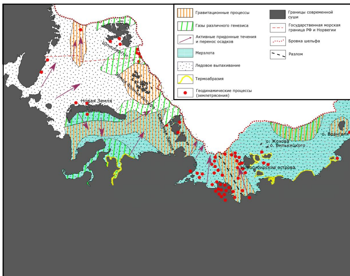
Рисунок 15. Картограмма опасных геологических процессов российской Арктики.
