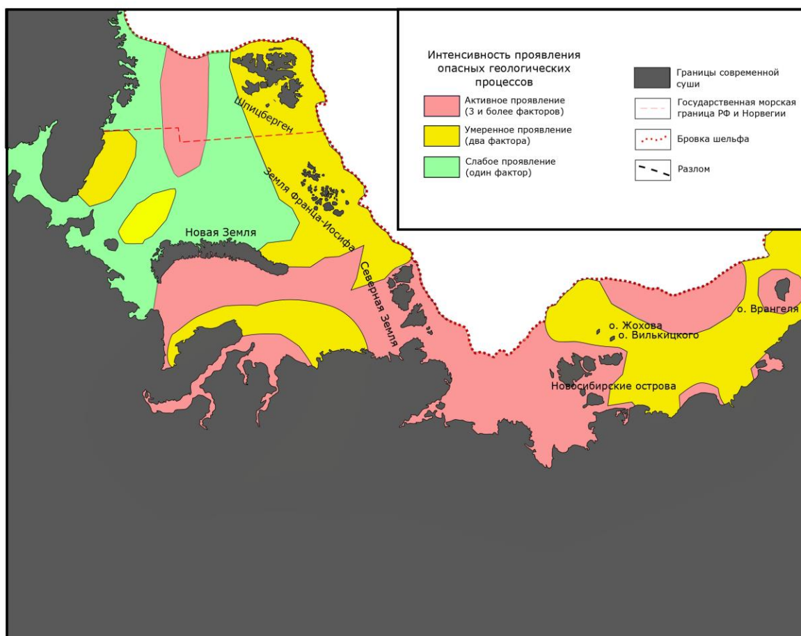
Рисунок 16. Картограмма районирования полярных морей России по характеру проявления опасных геологических процессов.
