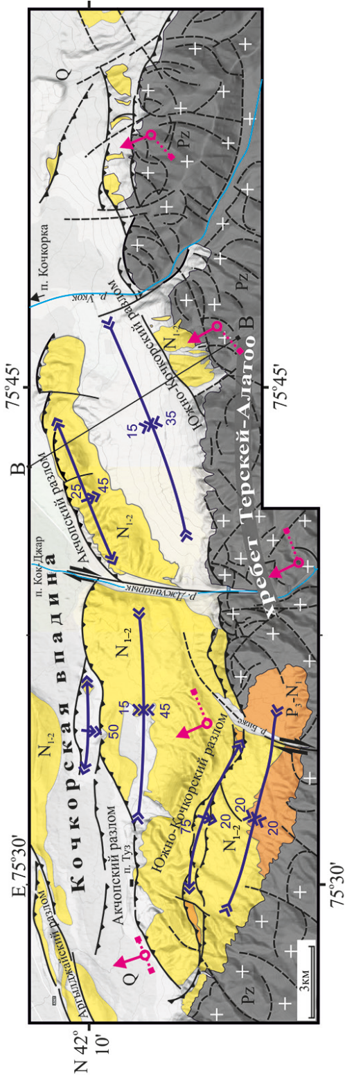
Рис. 4. Структурно-геологическая схема переходной зоны Кочкорской впадины — хр. Терсей-Алаато, по (Przhiyalgovskii et al., 2018) с дополнениями. Условные обозначения: см. рис. 2
