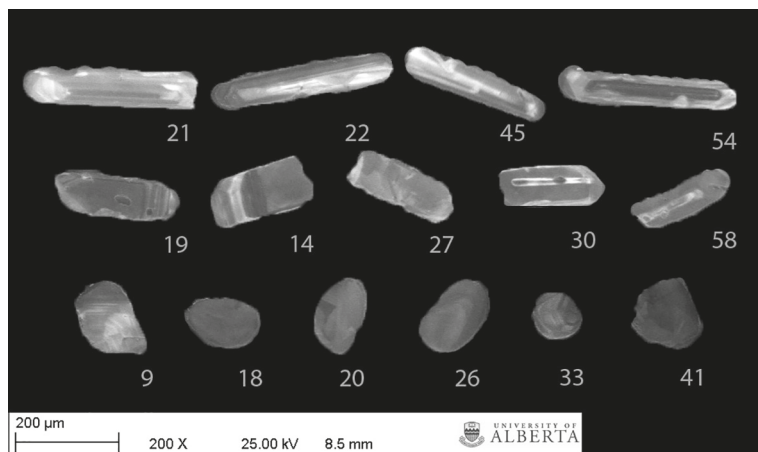
Рис. 3. Катодоллюминесцентное изображение обломочных цирконов из нижнекембрийских песчаников Уджинского поднятия
