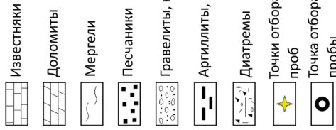
Рис. 1. Схема корреляции раннекембрийских разрезов севера Сибирской платформы (Гусев и др., 2016; Сметаникова и др., 2012)
