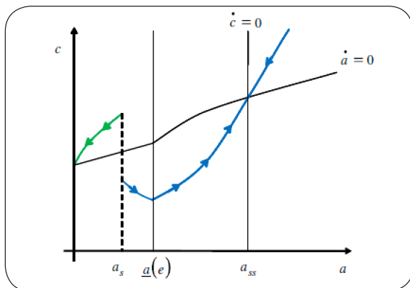
Рис. 1. Оптимальные траектории потребления ( c ) и богатства ( a ) агентов
