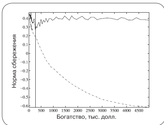
Рис. 2. Норма сбережения индивидов с наибольшими трудовыми способностями
