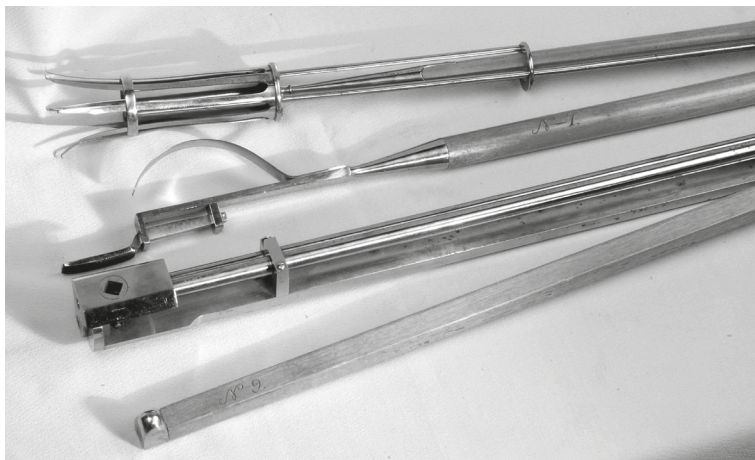
Рис. 2. Модель «машины для заделывания винтами раковин, открывающихся в каналах орудий». Александровский пушечный завод, Петрозаводск. 1835. Масштаб 1:2–3. Из коллекции Горного музея
