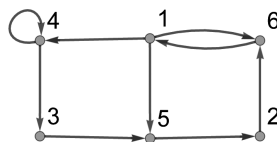
Рис. 2. Граф \mathcal{B}_6 .
