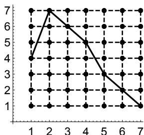
Рис. 1. График отображения f в случае n = 3 .
