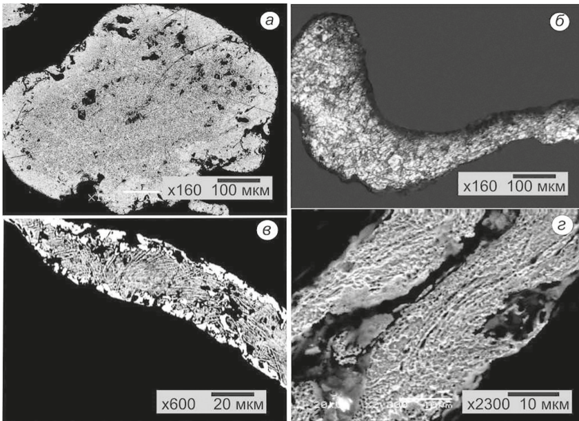
Рис. 3. Внутреннее строение россыпного золота: а, б — перекристаллизованные структуры; в, г — структуры пластических деформаций
