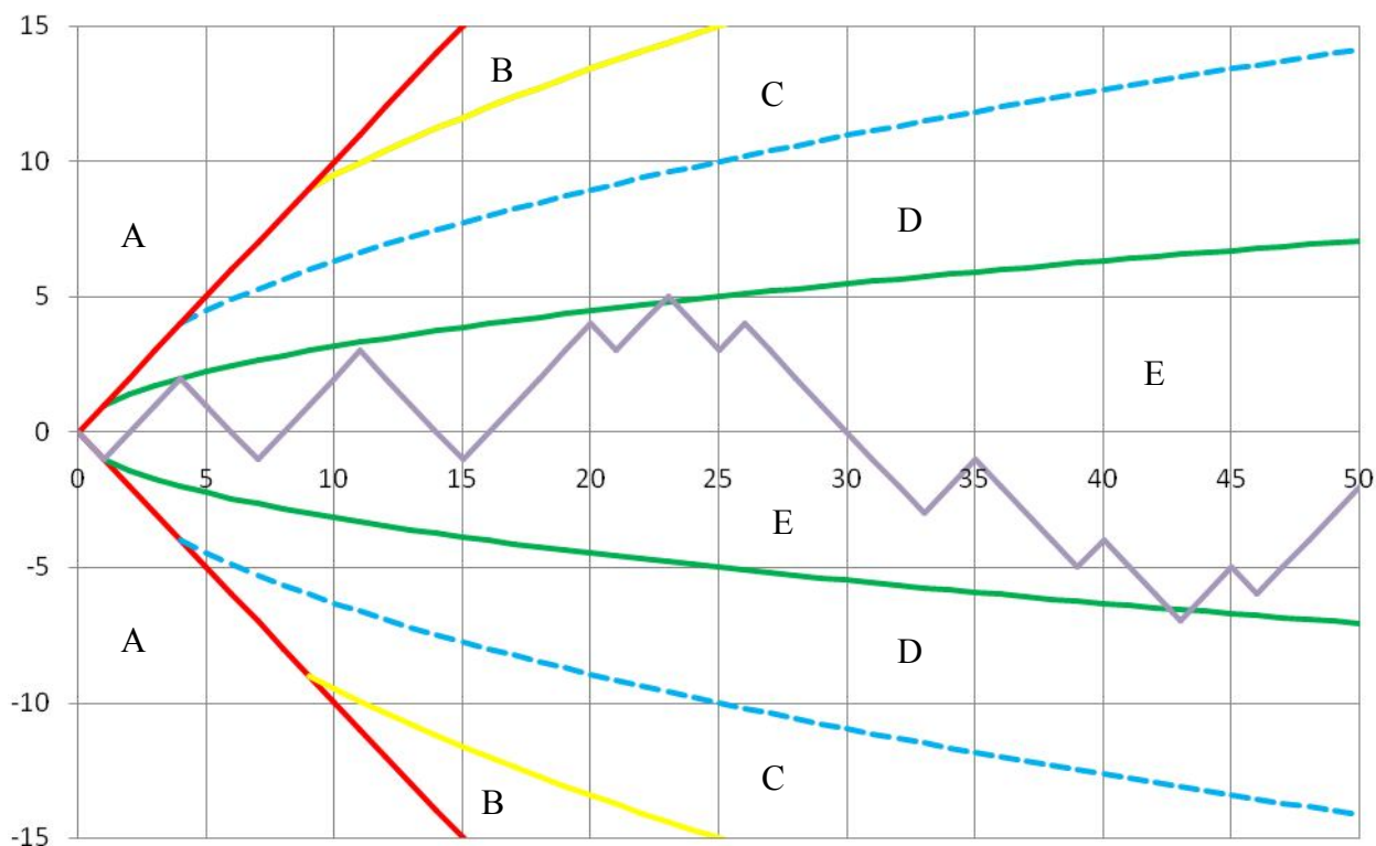
Рис.35. Зависимость выигрыша от числа испытаний при равенстве вероятностей успеха и неудачи (получена в компьютерном эксперименте). Линии разделяют зоны, где точке графика находится: А — невозможно; В — практически невозможно (отклонение превзошло три среднеквадратических); С — крайне удивительно (отклонение превзошло два среднеквадратических); D — несколько удивительно (отклонение превзошло среднеквадратическое); E — совершенно нормально.
