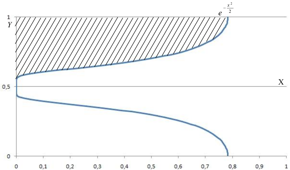
Рис. 40. График функции X = e^{-\frac{x^2}{2 \cos^2(\pi Y)}} .
