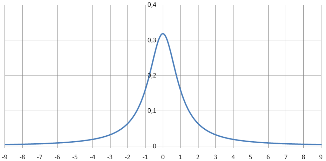
Рис. 30. Плотность вероятности распределения Коши.
