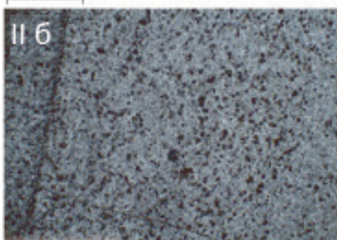
Рис. 3. Часто встречаемые частицы в породах кремнистого горизонта
