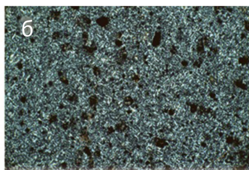
Рис. 4. Микрочастицы на оолитах и пеллетах фосфата в породах кремнистого горизонта
