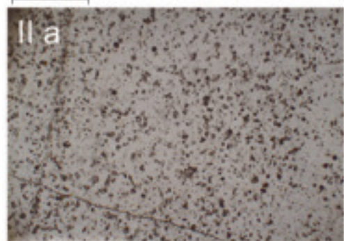
Рис. 3. Часто встречаемые частицы в породах кремнистого горизонта
