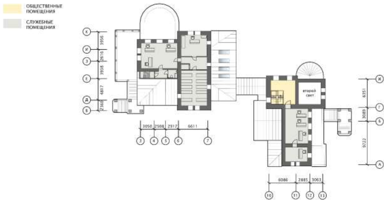
Рис. 3.10 План 4 этажа
