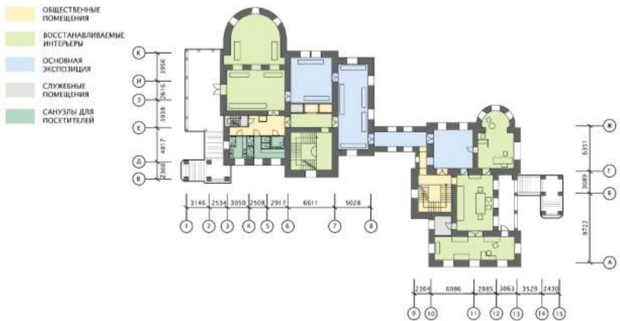
Рис.3.8 План 2 этажа
