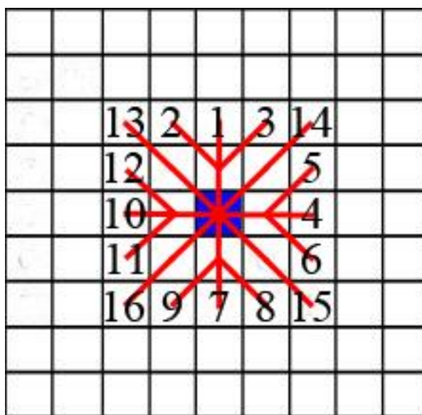
Рис. 1.3. Второй этап распространения волны
