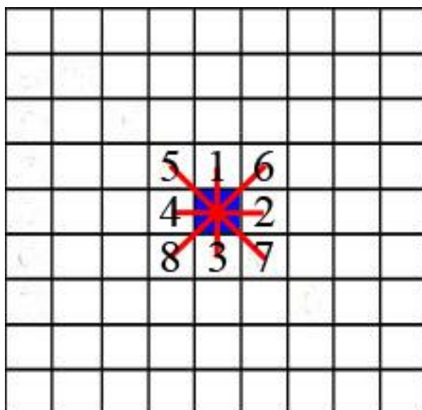
Рис. 1.2. Первый этап распространения волны
