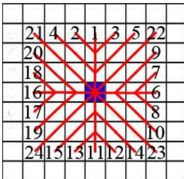
Рис. 1.4. Третий этап распространения волны
