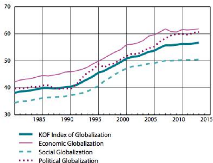
Рис. 5 – Индекс мировой глобализации KOF за период 1980-2013 гг.
