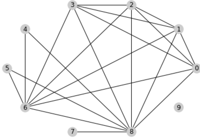
Рис. 1: Пороговый граф.
